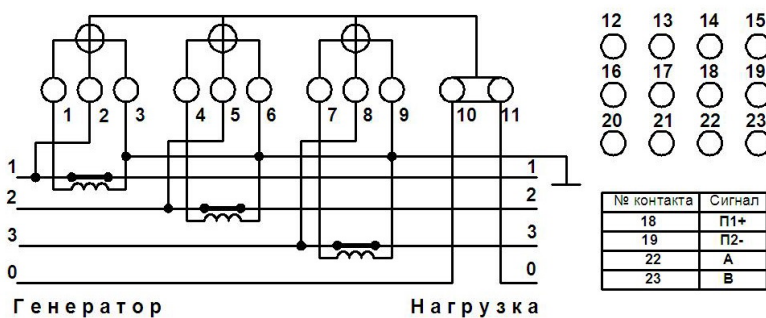
Рисунок 5. В корпусе B04, трансформаторное подключение
