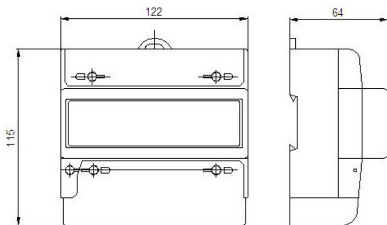
Рисунок 3. Корпус R02
