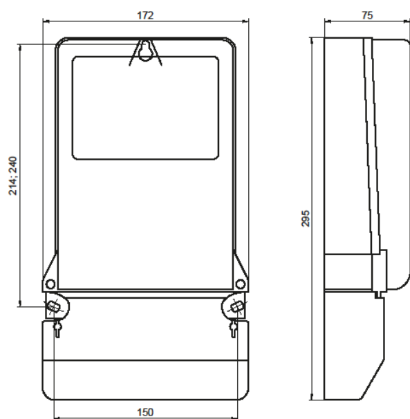
Рисунок 2. Корпус B04
