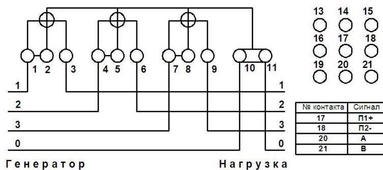
Рисунок 4. В корпусе B04, непосредственное подключение.
